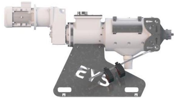
Opsiyonel Paslanmaz Çelik Gövde Optional Stainless Steel Body Available
