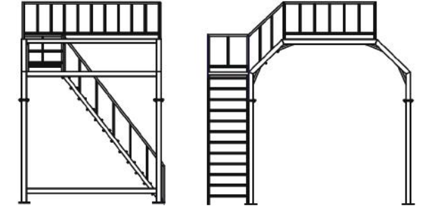
Modüler Galvanizli Platform (SP600 ve daha büyük modeller için) Modular Galvanized Platform (For SP600 and bigger models)
