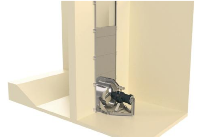
Kaset Tip Sirkülasyon Kaidesi – Z Tip Circulation Frame with Z Rails
