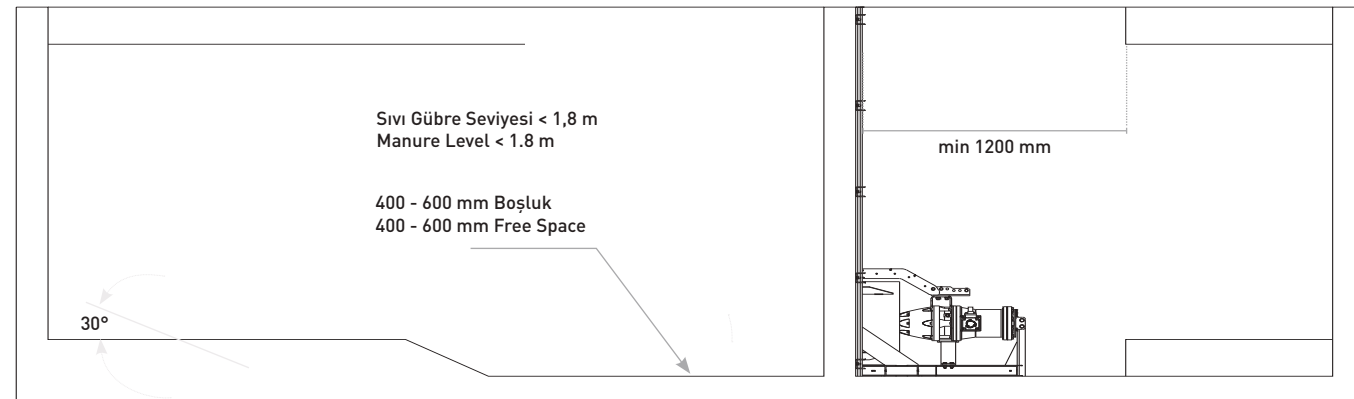
Dalgıç karıştırıcıların slalom tip havuzlar ve kanallar içerisindeki yerleşimi Positioning of submersible mixers in slalom type pits and in corridors
