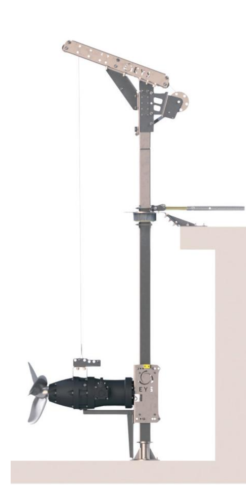
Standart Yerleşim Standart positioning
