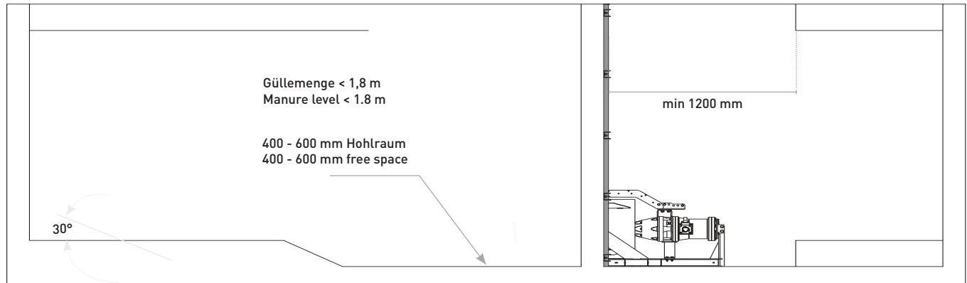
Positionierung von Tauchmotorrührwerken in Slalomgruben und in Gängen Positioning of submersible mixers in slalom type pits and in corridors
