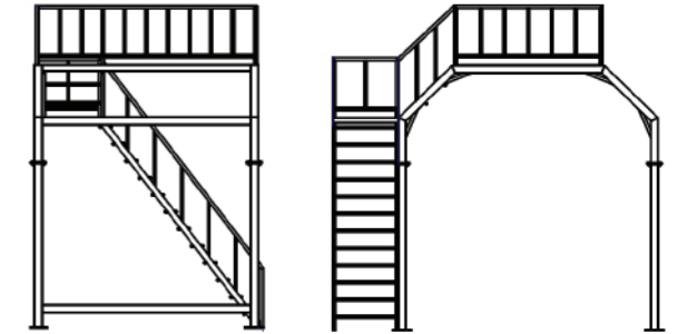
Modüler Galvanizli Platform (SP600 ve daha büyük modeller için) Modular Galvanized Platform (For SP600 and bigger models)
