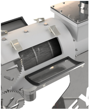
Gövde üzerinde çift gözetleme kapağı Observation window on both sides of separator body
